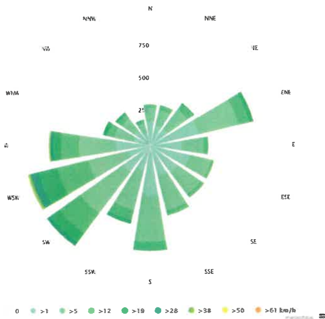
Roza vânturilor
